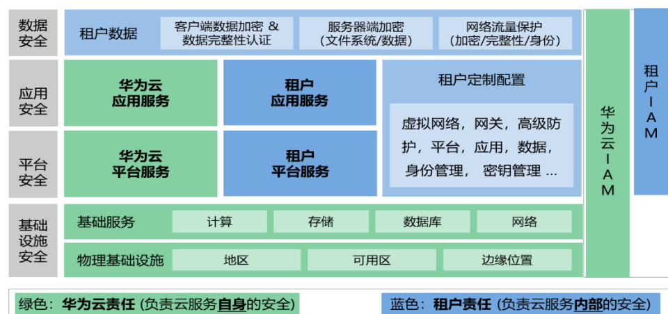
图2-1 华为云安全责任共担模型
