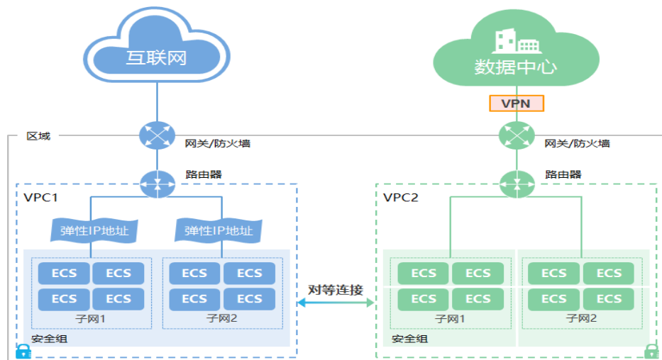
图6-1 华为云 VPC 架构简图
