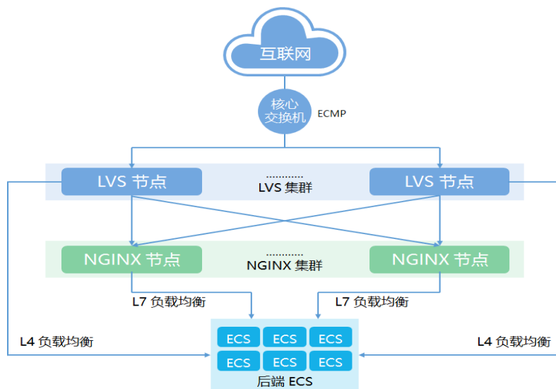
图6-2 华为云 ELB 组网图
